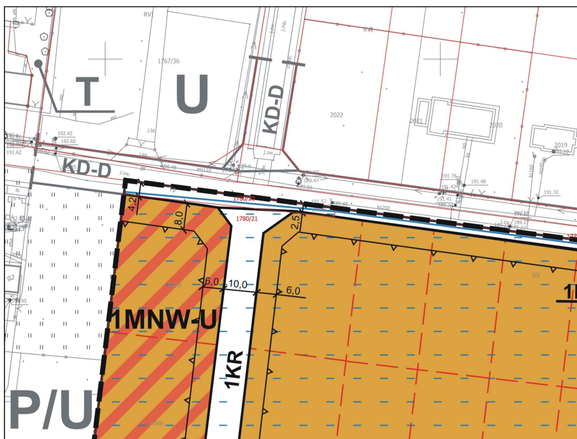
Rysunek planu - fragment nr 1
